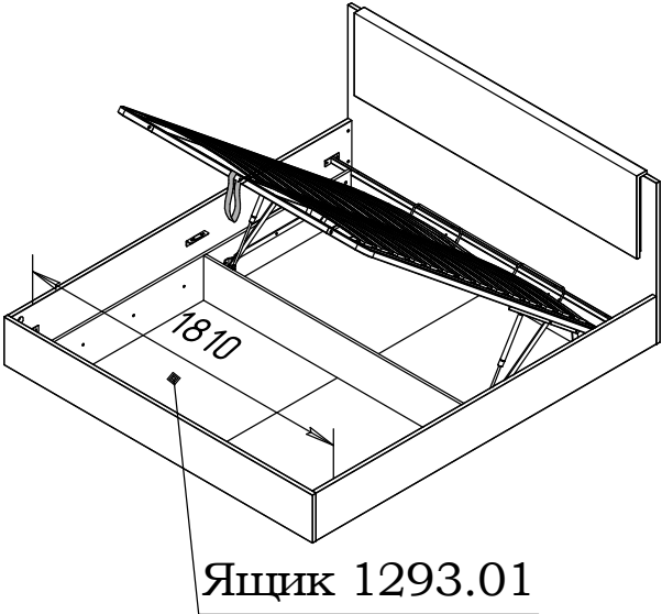
Кровать 61.202.00.00-01
