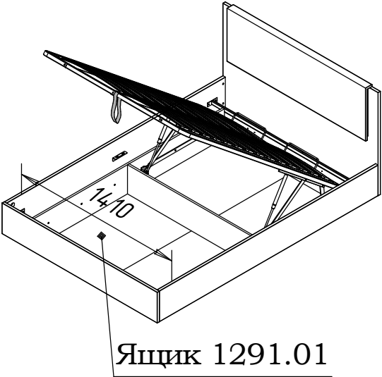
Кровать 61.202.00.00-01
