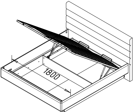
Кровать 46.283.00.00-02 (-03)
