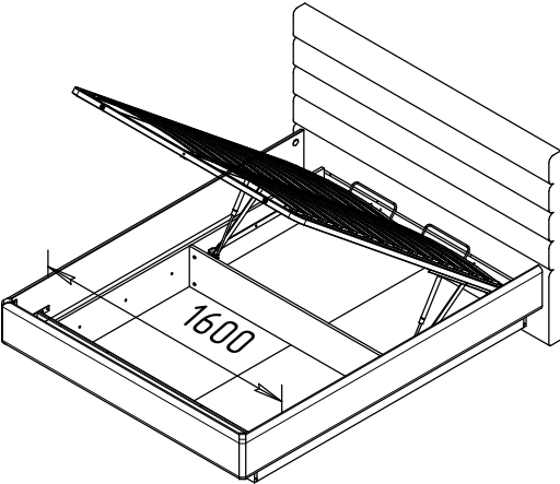
Кровать 46.282.00.00-02 (-03)
