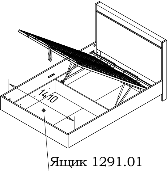
Кровать 62.200.00.00-01
