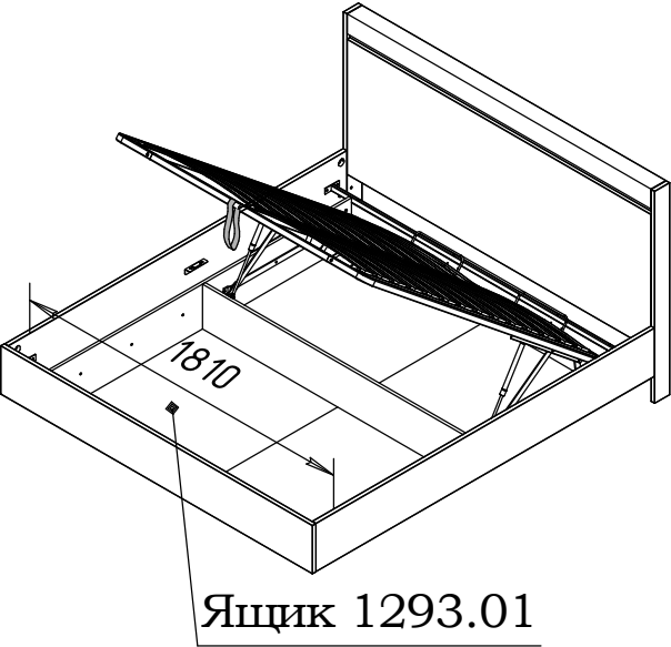
Кровать 62.202.00.00-01
