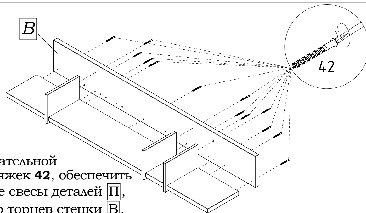
Схема полки 53.050.00.00 (вид сзади)
