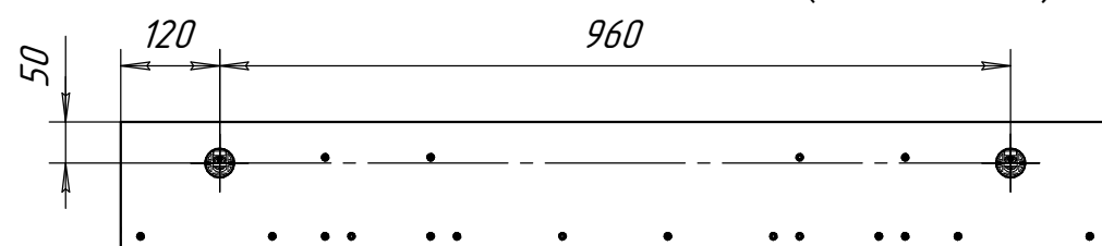
Схема полки 53.050.00.00 (вид сзади)
