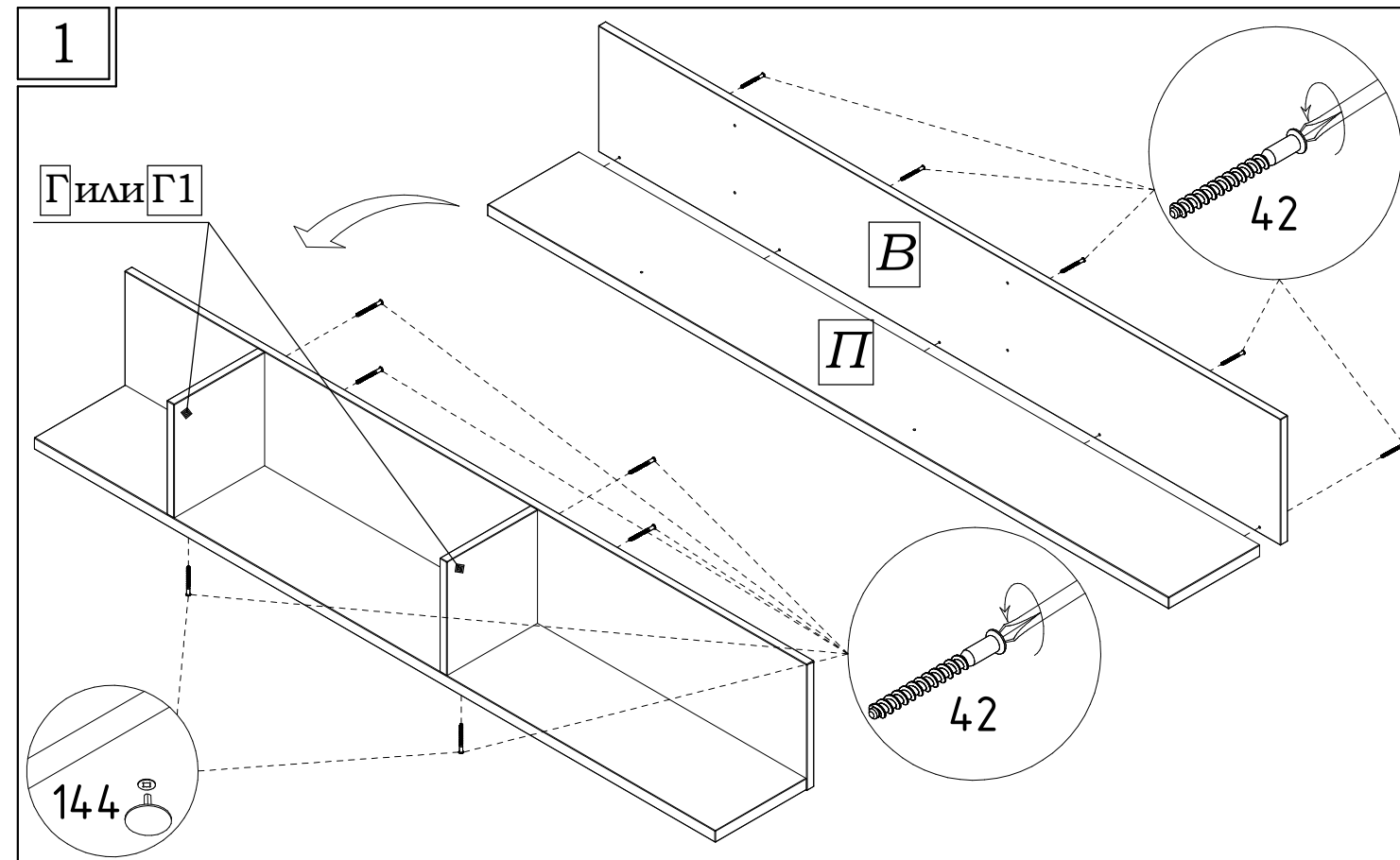
Схема полки 51.342.00.00 (вид сзади)
