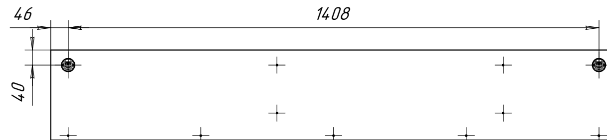
Схема полки 51.342.00.00 (вид сзади)
