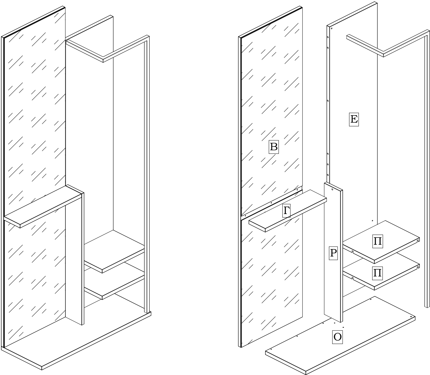
Вешалка 64.060.00.00.00
