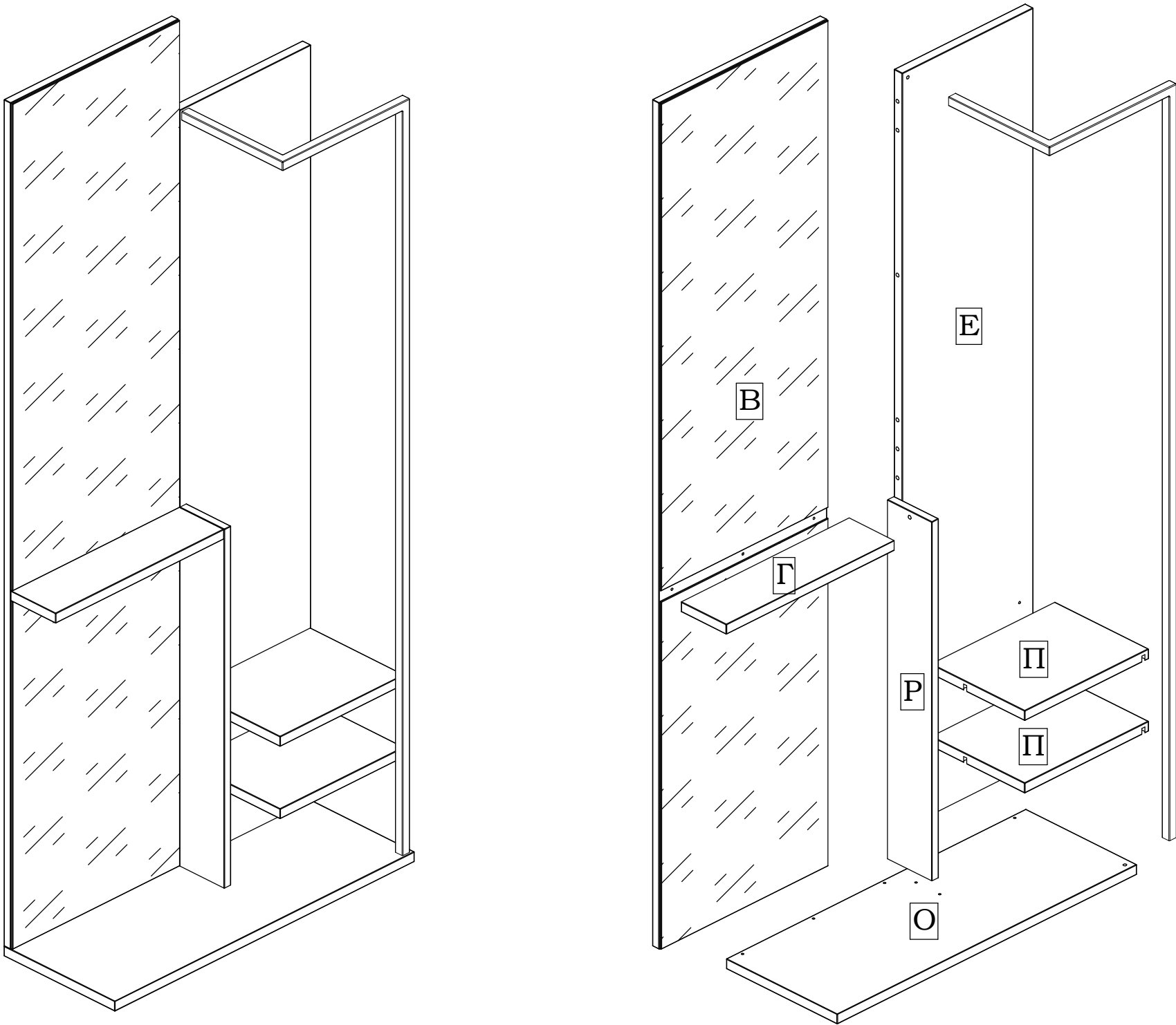
Вешалка 64.060.00.00.00
