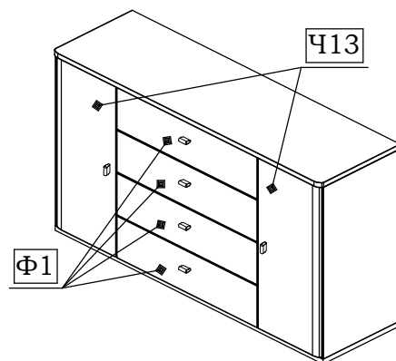
Тумба 46.511-01
