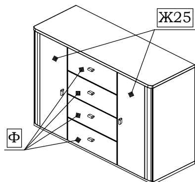
Тумба 46.509
