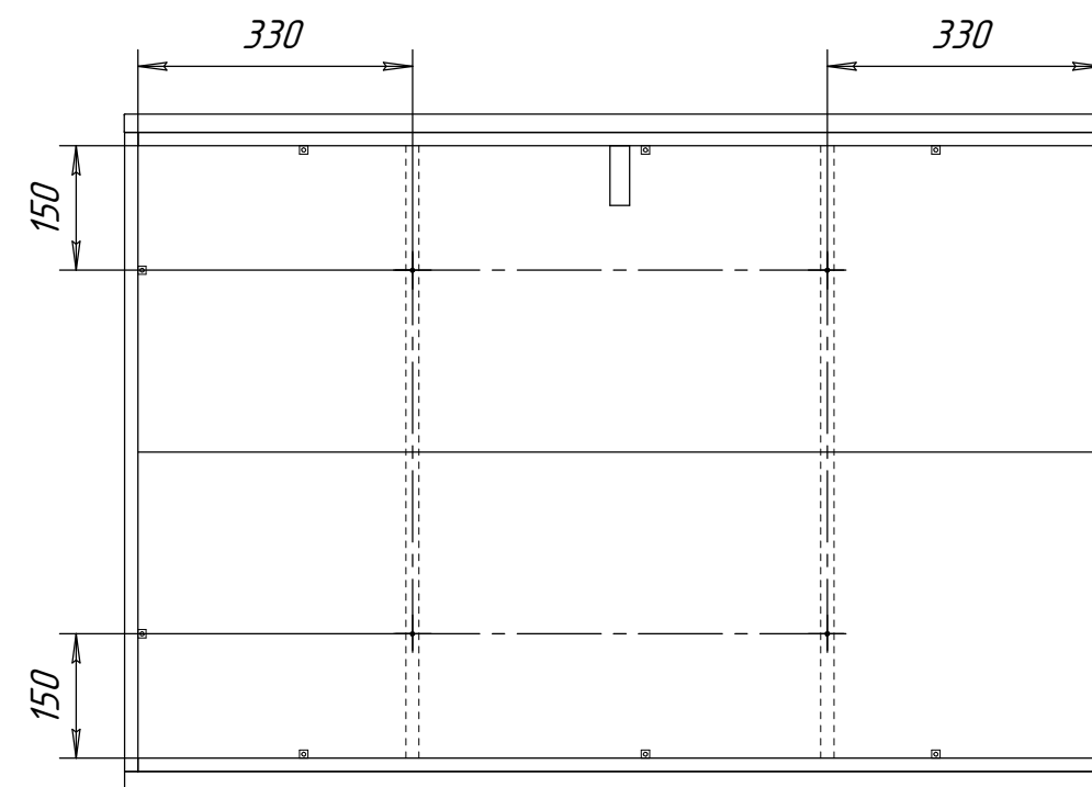
Вид сзади
