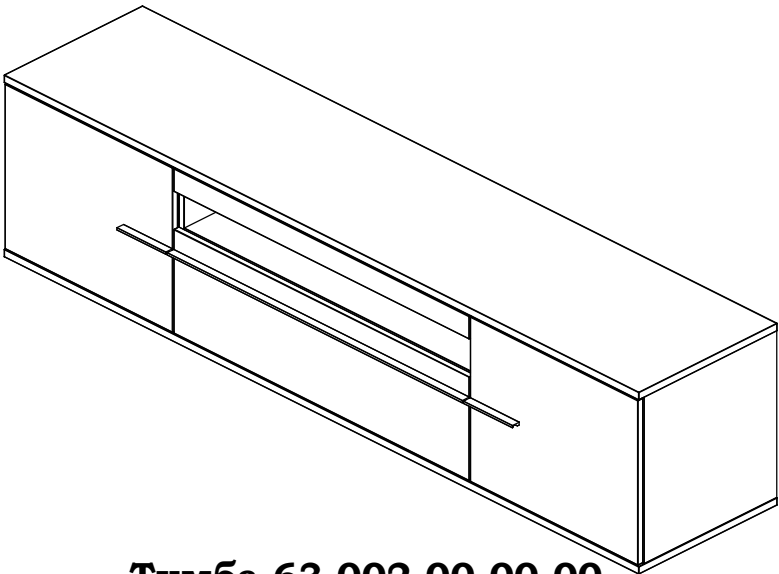
Тумба 63.002.00.00.00
