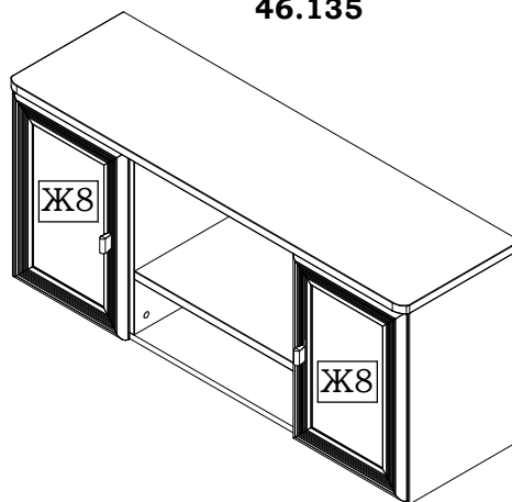
Шкаф настенный 46.135
